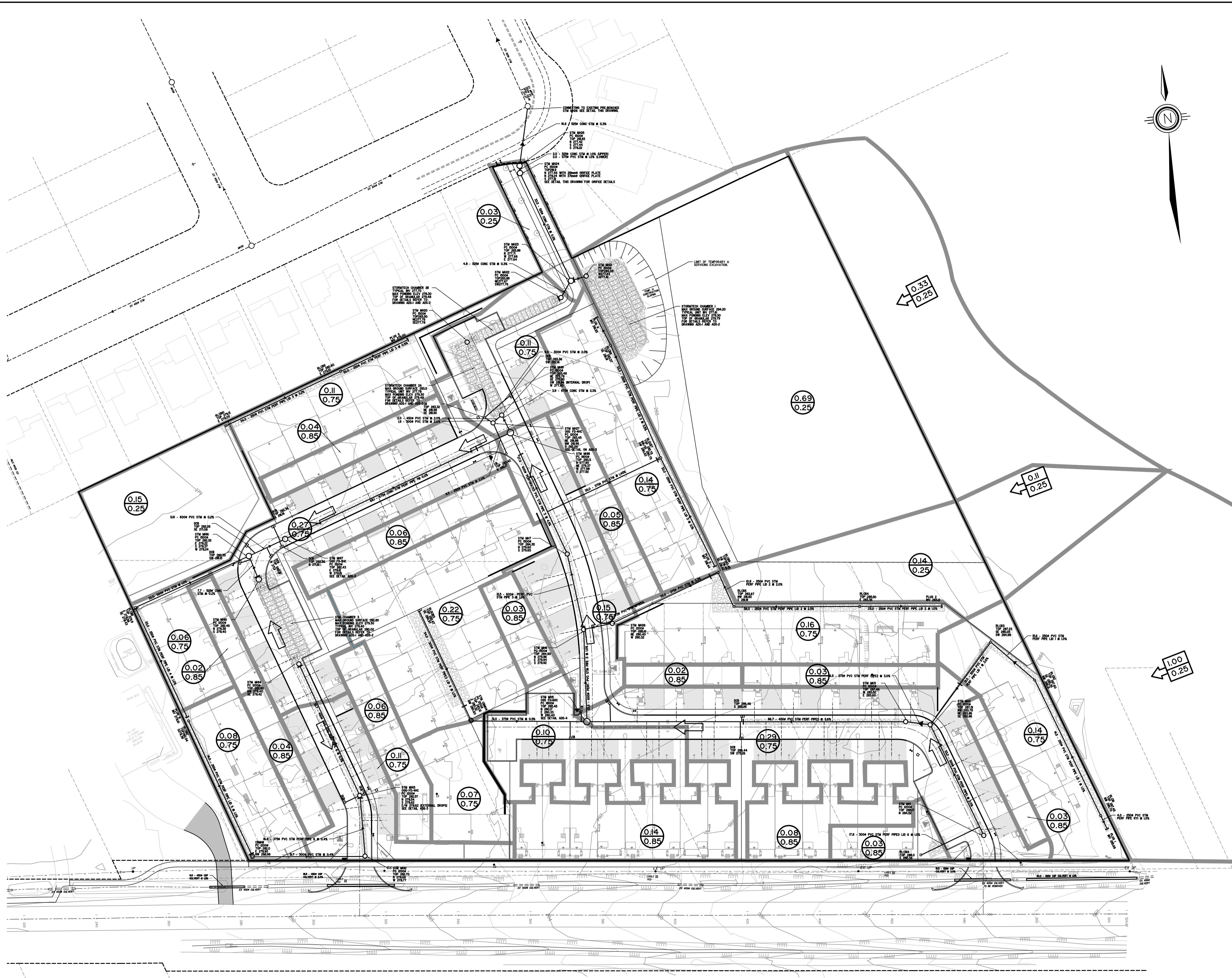
KEYMAP N.T.S.
